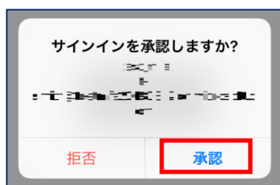
【iOS 画面】
